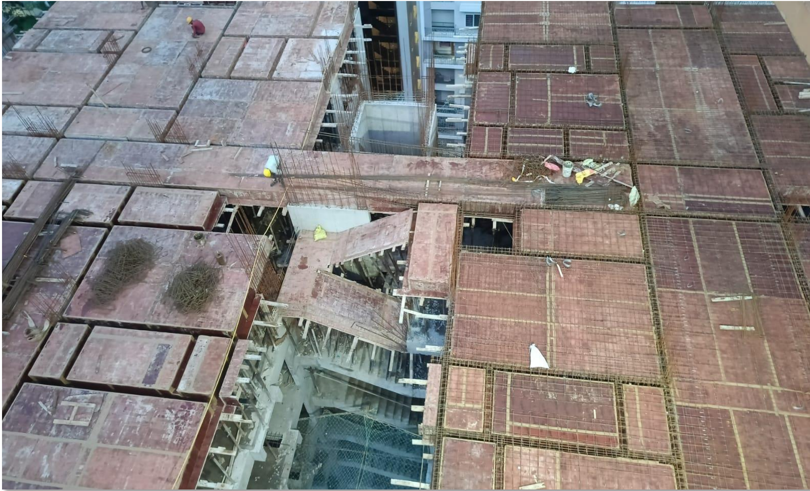
Pour 1 13 th floor roof shuttering completed.
